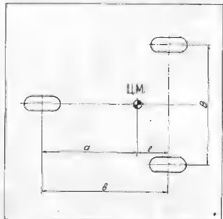
Рис.5. Параметры шасси с носовой опорой
